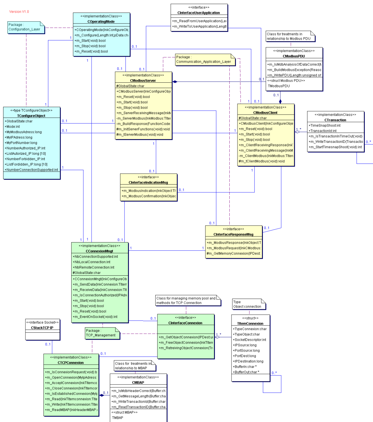
图 22: 类的示意图
